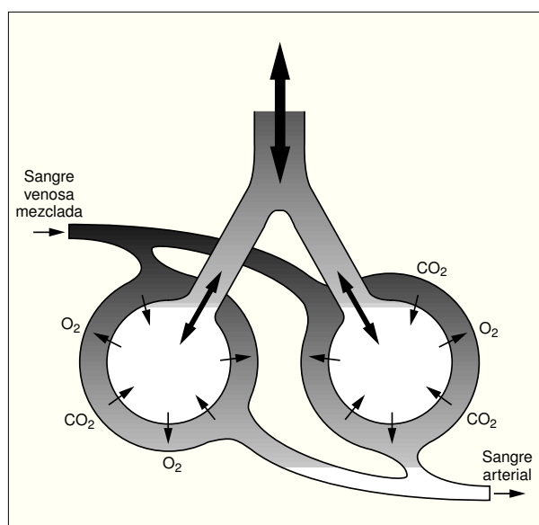
Figura 1. Unidad funcional pulmonar. Esquema de intercambio de gases entre el compartimento aéreo y el compartimento vascular.
